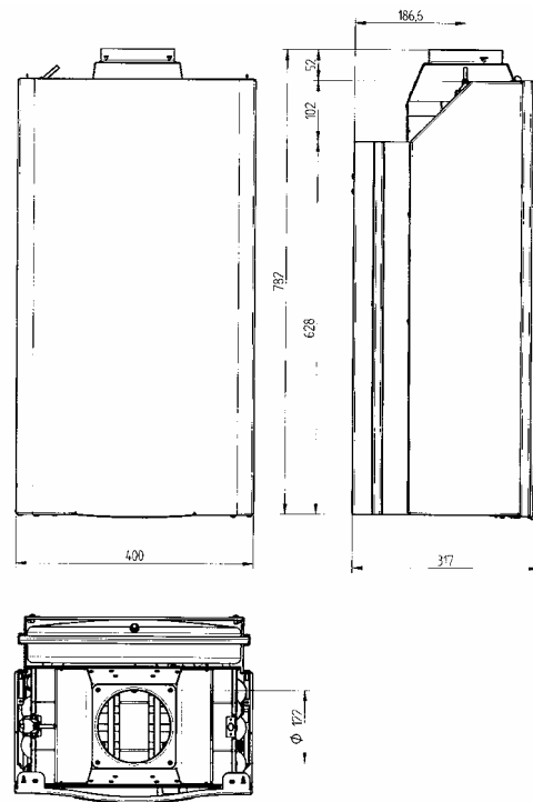
Модель 1.140 Ø = 112 мм
